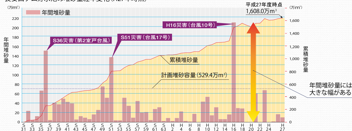
長安ロダム貯水池の堆砂量経年変化 (H27年時点)
