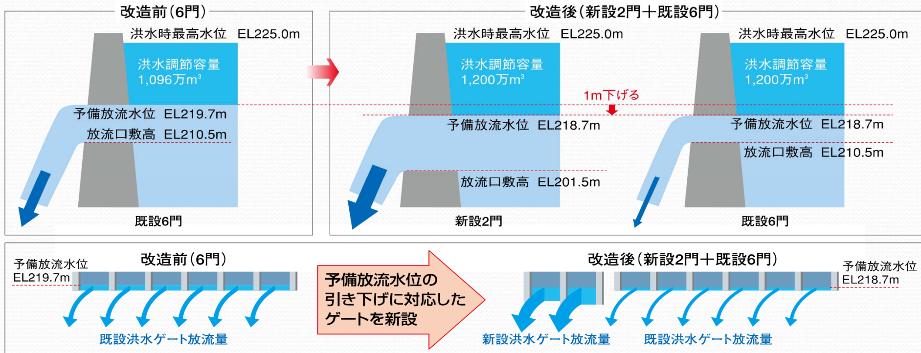
■ゲート放流イメージ図
