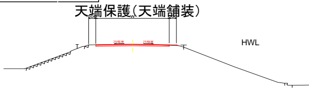
断面図(石手川3.0Kp)
