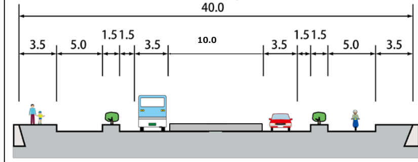
【標準断面図 (副道設置部 (暫定2車線))】 (単位 m)
