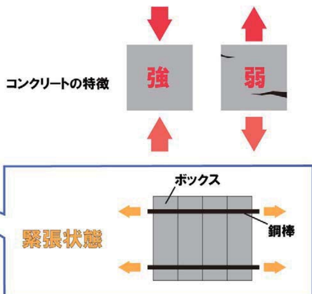
コンクリートブロックを用いて鋼棒を緊張している様子
