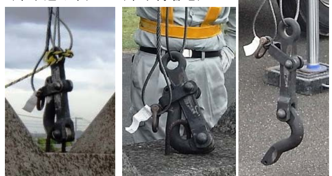
①ロック状態 ②ストッパー解除 ③フック開放 (吊り込み中) (吊り荷着地)
