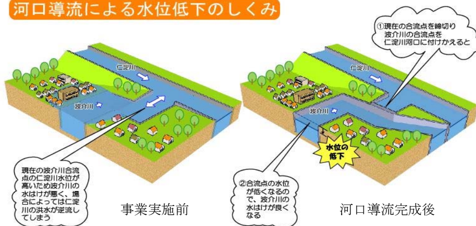
図 7 波介川河口導流による水位低下のしくみ
