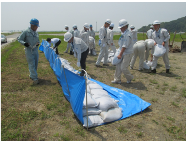
越水対策 (改良積土のう工)
