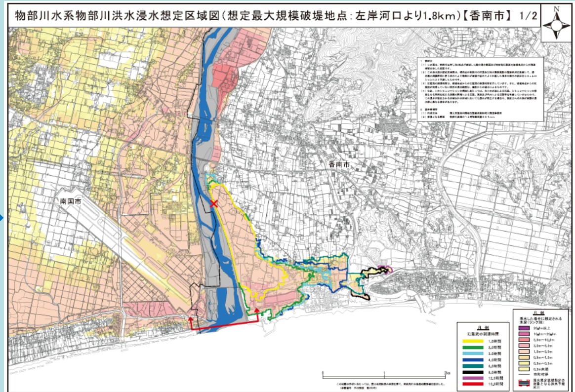
氾濫流の到達時間を表示した浸水想定区域図
