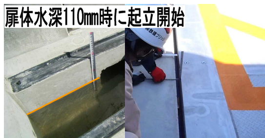
手動による全起立（堤内側）状況
