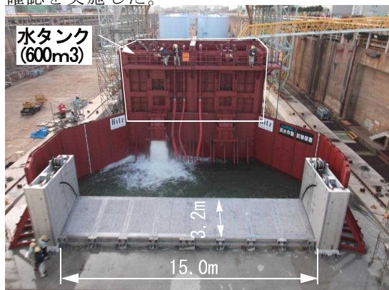
図－8 工場試験装置
