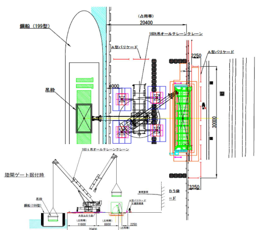
図-11 現地据付要領図
