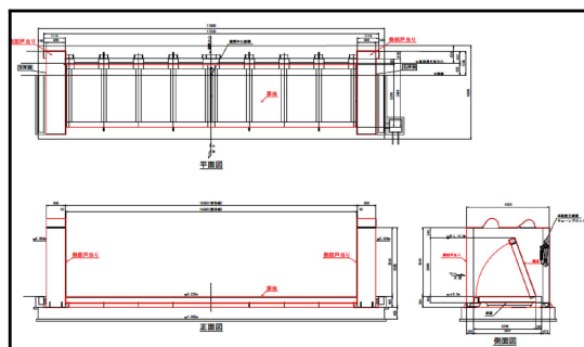
図-6 陸閘ゲート設備一般図
