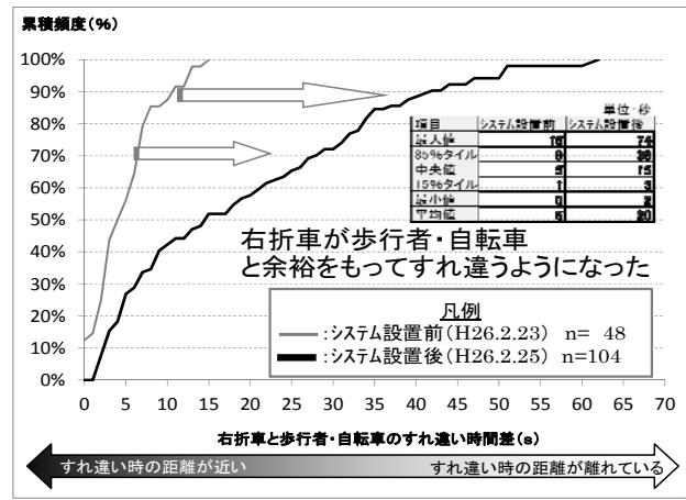
図-8 すれ違い時間差の変化 (河ノ瀬交差点)
