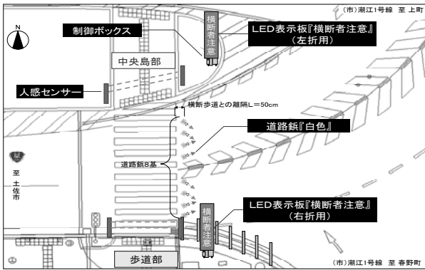
図-4 システム配置図(河ノ瀬交差点)
