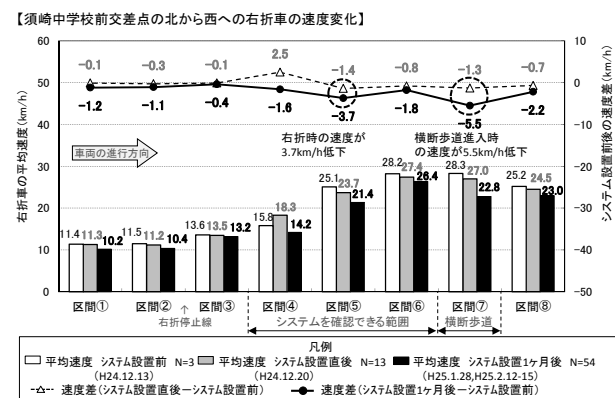
図-7 ビデオ調査の画像解析による右折時の速度変化
