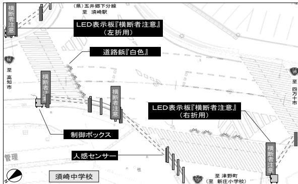
図-5 システム配置図(須崎中学校交差点)
