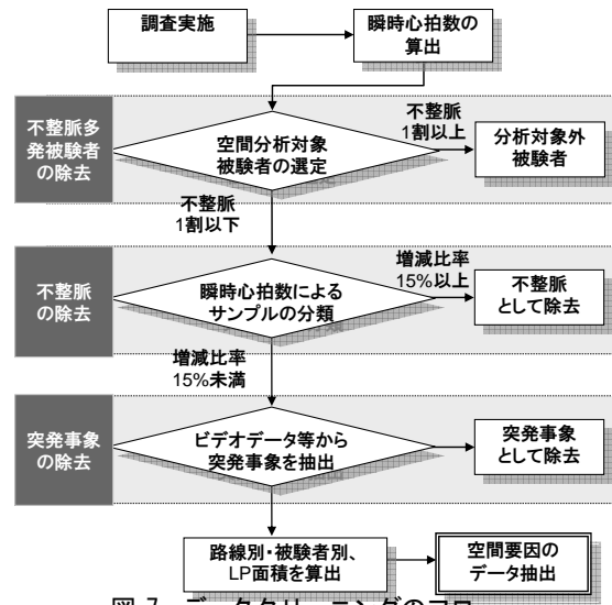
図-7 データクリーニングのフロー
