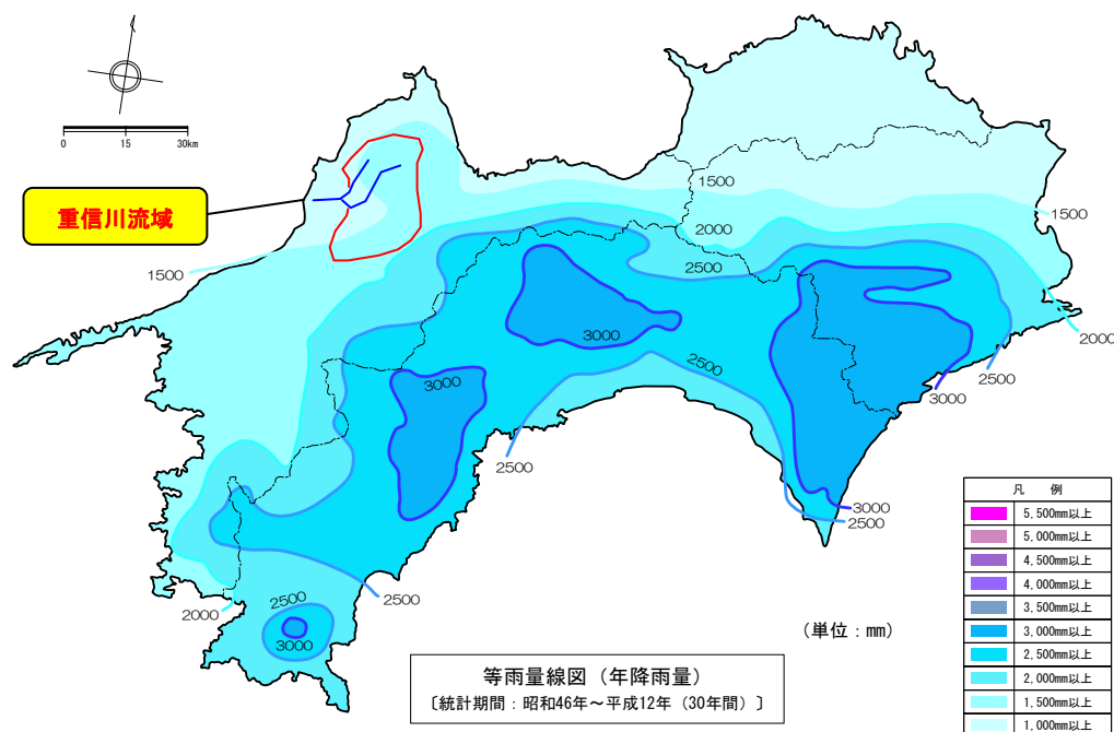
図 1.4.1 四国の年平均降水量分布
