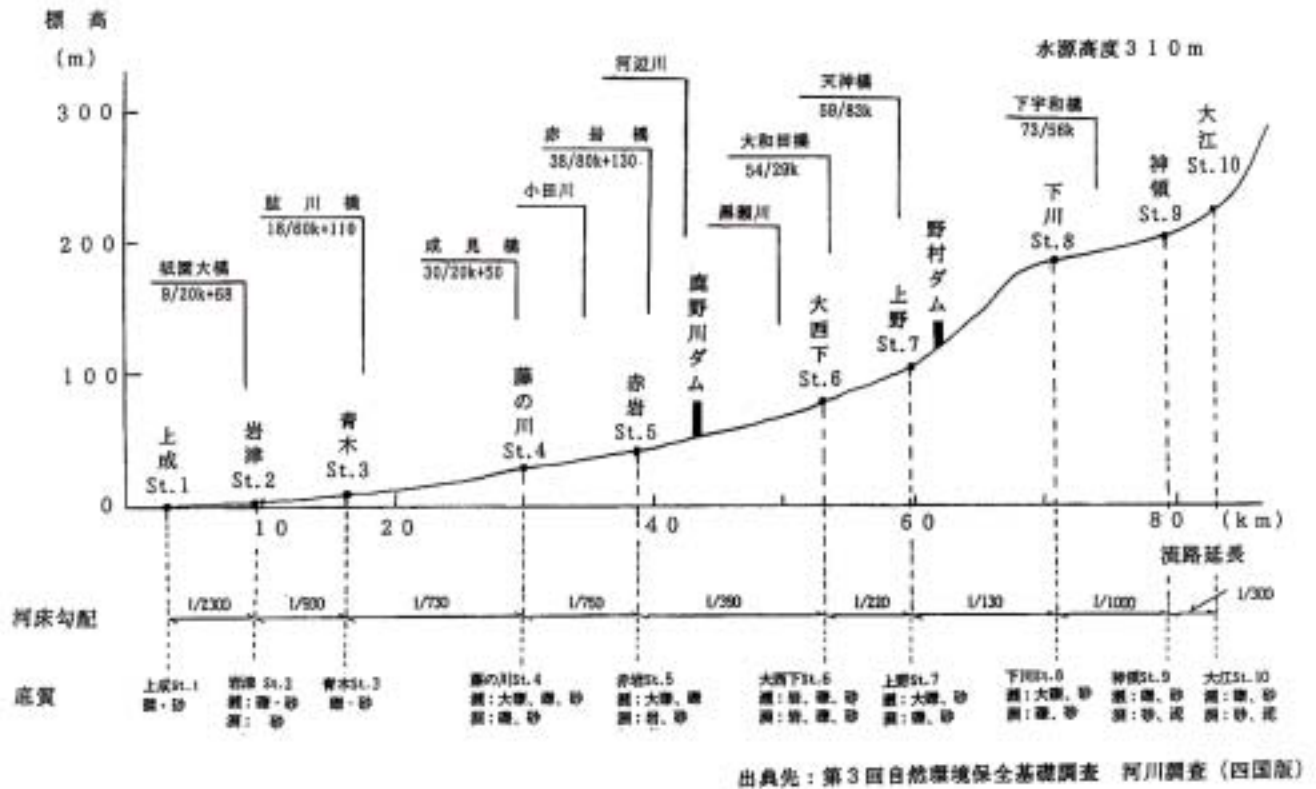
図 8-1 肱川河床縦断勾配図
