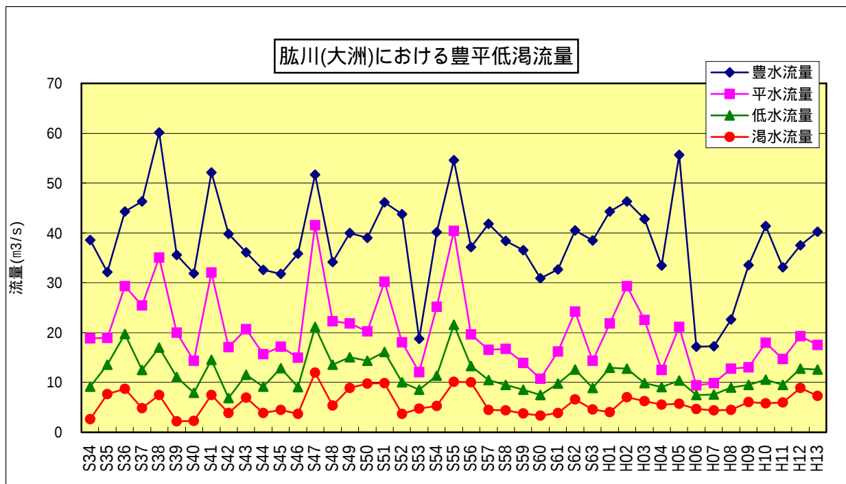
図 6-1 肱川の流況
