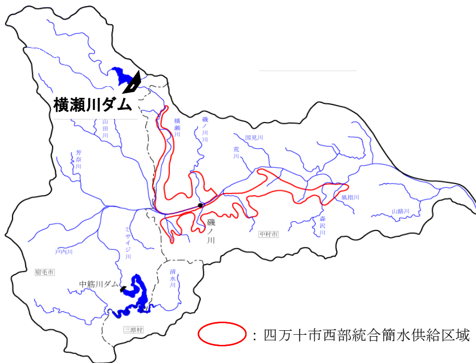
図 2-5-1 四万十市西部統合簡易水道供給区域
