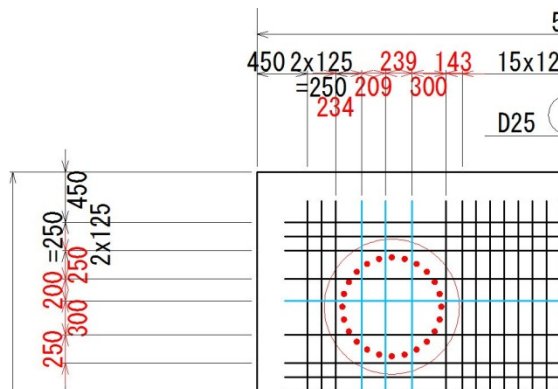
②修正(鉄筋間隔を調整)
