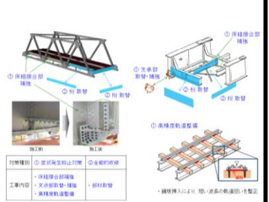
大規模改修工事の内容【鋼橋】
