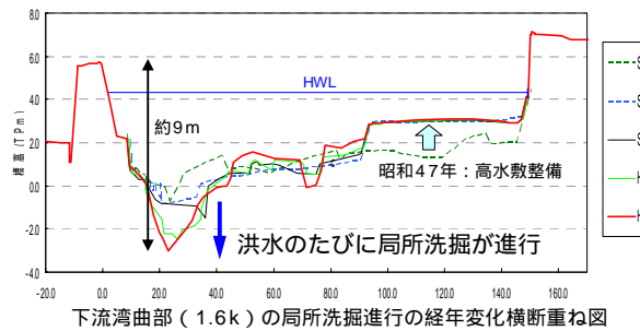
下流湾曲部（1.6k）の局所洗掘進行の経年変化横断面重ね図
