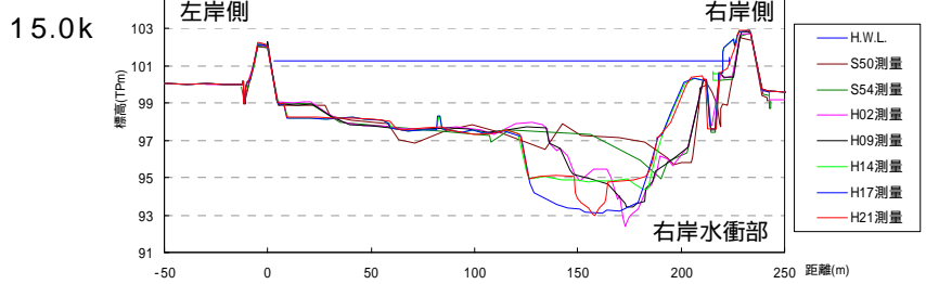
河床低下区間の水衝部（14.6k、15.0k付近）の経年変化横断重ね図
