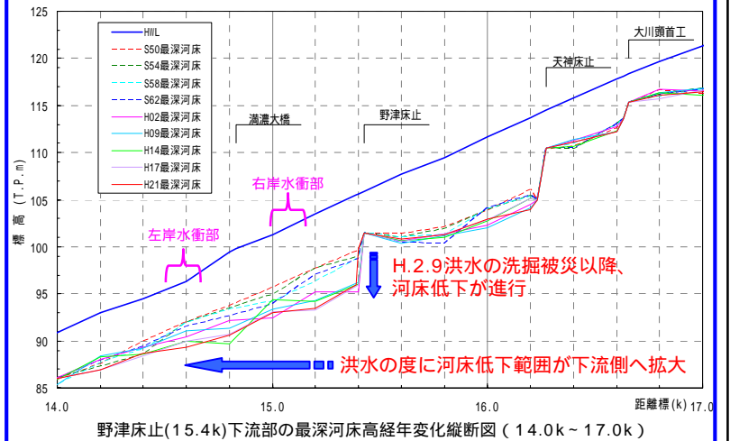
野津床止(15.4k)下流部の最深河床高経年変化縦断面図（14.0k～17.0k）
