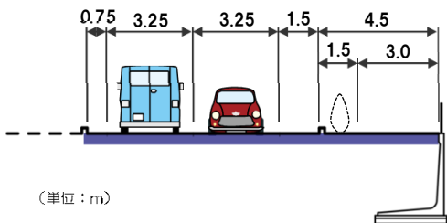
【標準断面図】(暫定2車線開通時)
