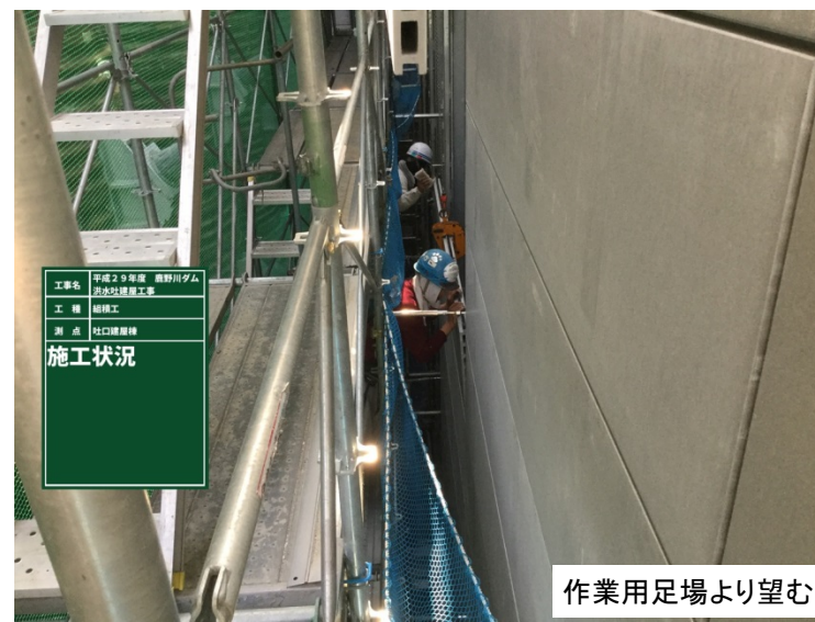
4月9日 吐口建屋棟押出し成形セメント板取付
