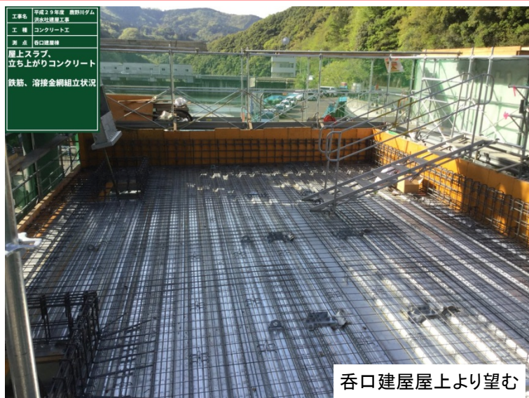
4月16日 呑口建屋棟屋上スラブコンクリート打設
