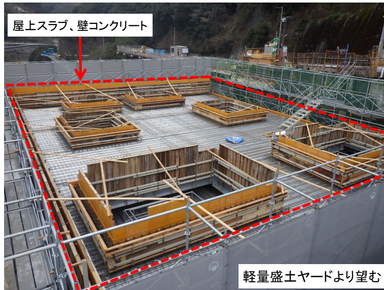
3月5日 屋上スラブ、壁コンクリート鉄筋・型枠組立
