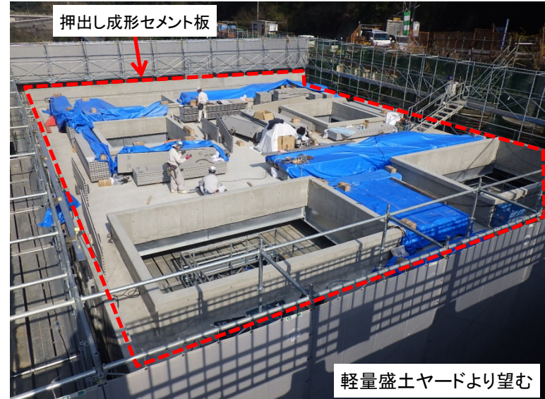
3月26日 押し成形セメント板取付
