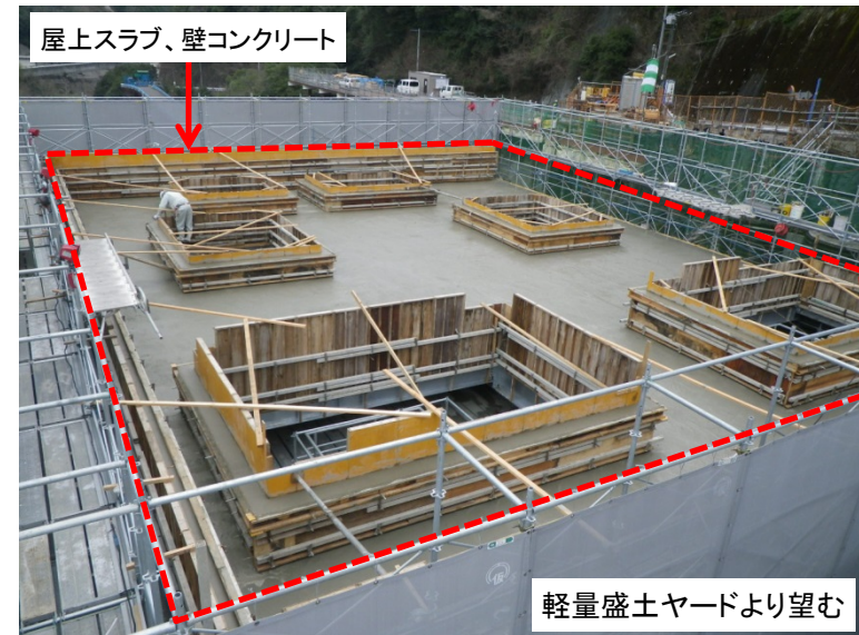
3月12日 屋上スラブ、壁コンクリート打設
