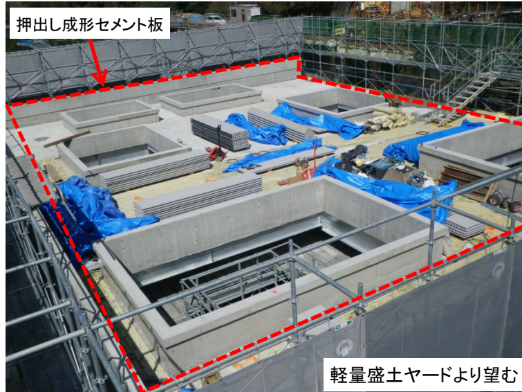
3月19日 押し成形セメント板取付
