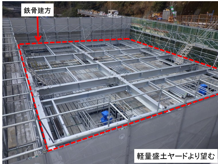
2月5日 吐口建屋棟鉄骨建方
