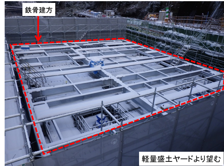
2月12日 吐口建屋棟鉄骨建方
