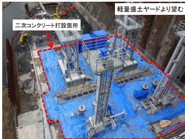
12月18日 二次コンクリート打設および養生
