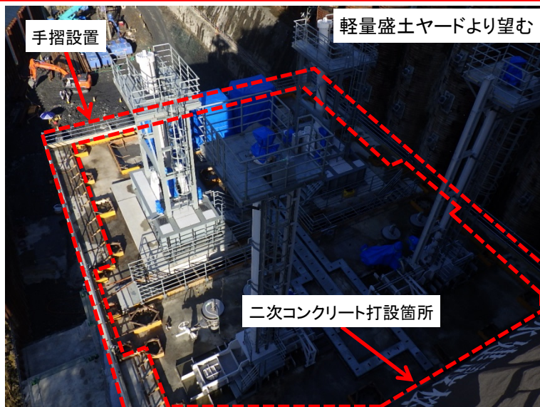
12月4日 手摺設置および二次コンクリート型枠組立
