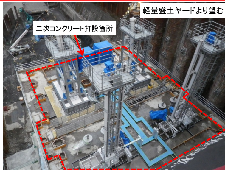
12月11日 二次コンクリート型枠組立
