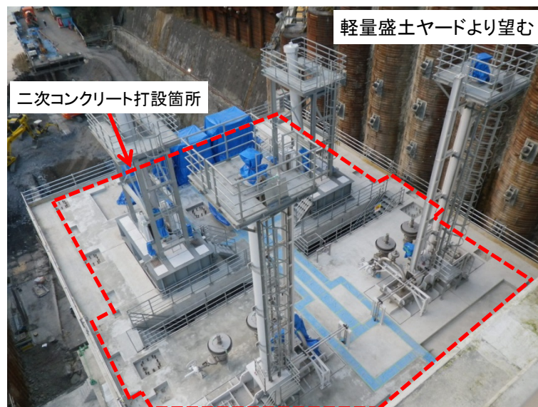
12月25日 二次コンクリート型枠解体
