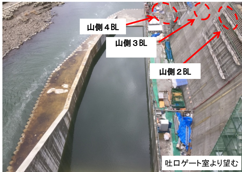
4月8日 山側2BL打設前清掃、3BL・4BLコンクリート打設
