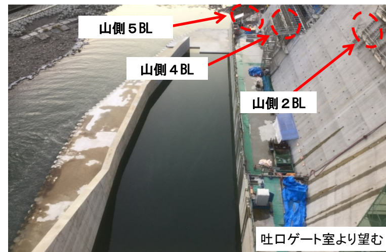
4月15日 2BL型枠組立、4BL・5BL打設前清掃
