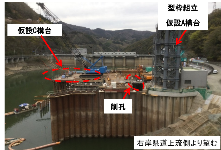
4月8日 呑口仮設(A・C)構台撤去、型枠組立、削孔
