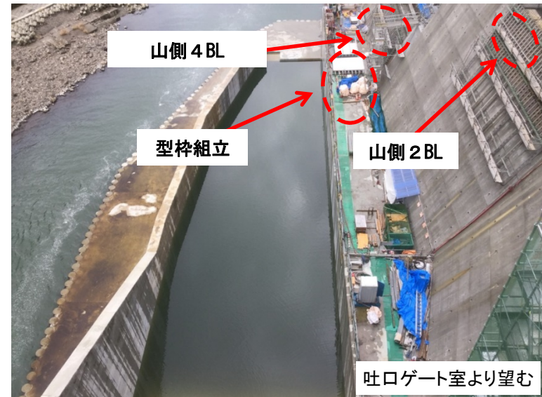
4月1日 山側2BL鉄筋組立、山側4BLコンクリート打設
