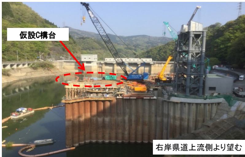
4月22日 呑口仮設(A・C)構台撤去、型枠組立
