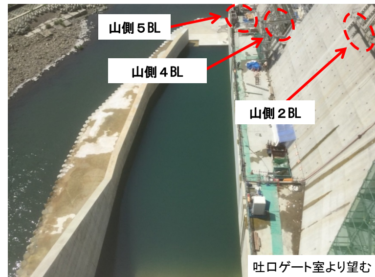
4月22日 山側2BL・5BL型枠組立、4BL水抜きパイプ設置
