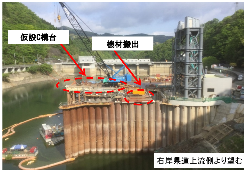
4月29日 呑口仮設(A・C)構台撤去、型枠組立、機材撤去
