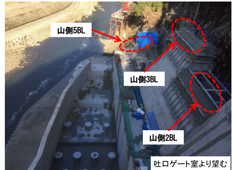
3月11日 山側2BL清掃、3BL鉄筋組立、5BLレイタンス処理
