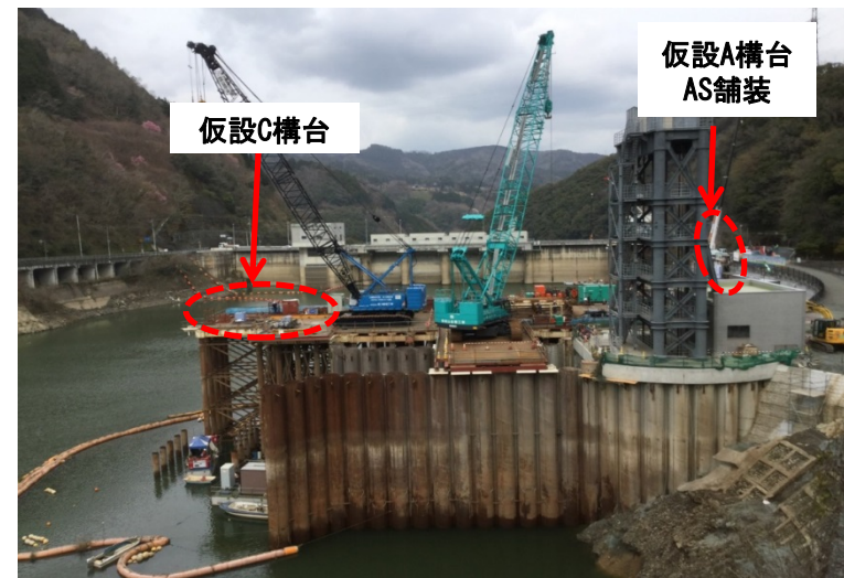
3月25日 仮設(A・C)構台撤去、AS舗装撤去
