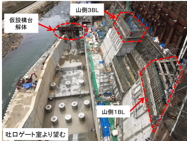
2月4日 山側1BLコンクリート打設、山側3BL型枠組立
