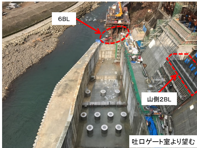
2月18日 6BL土留・仮締切撤去、山側3BL型枠組立
