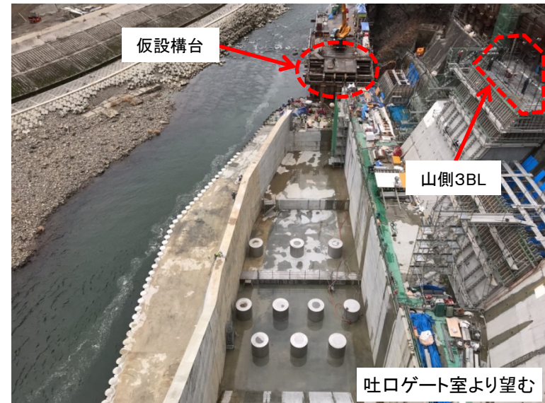
2月12日 山側3BL型枠組立、仮設構台解体
