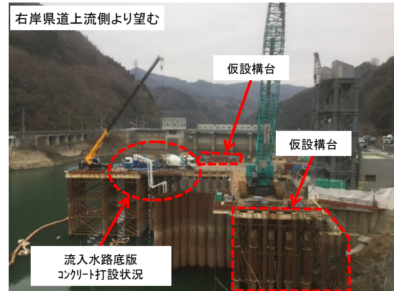
2月25日 水中コンクリート打設、仮設構台解体
