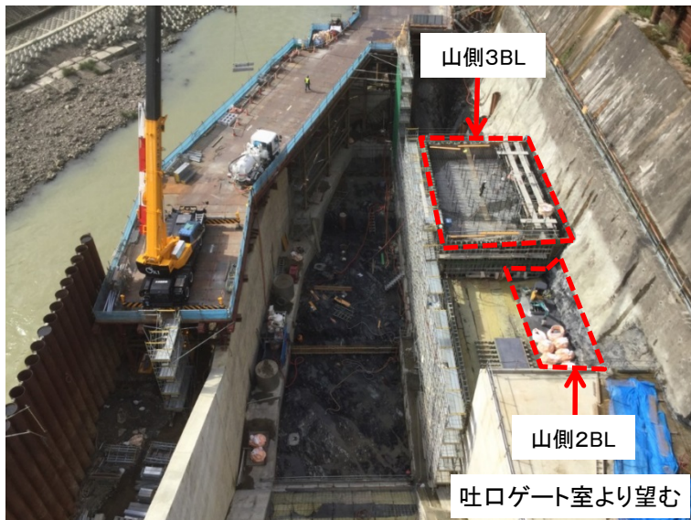
10月15日 山側2BLモルタル撤去、山側3BL鉄筋組立
