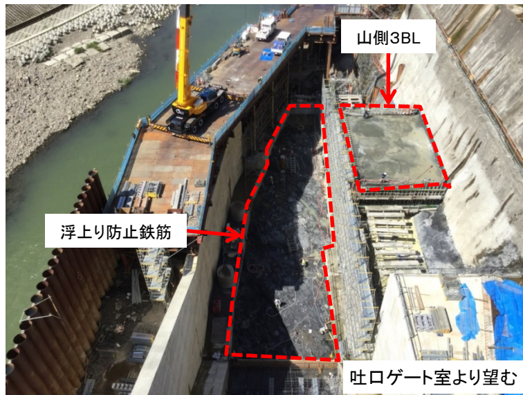
10月1日 山側3BLレイタス処理、浮上り防止鉄筋設置
