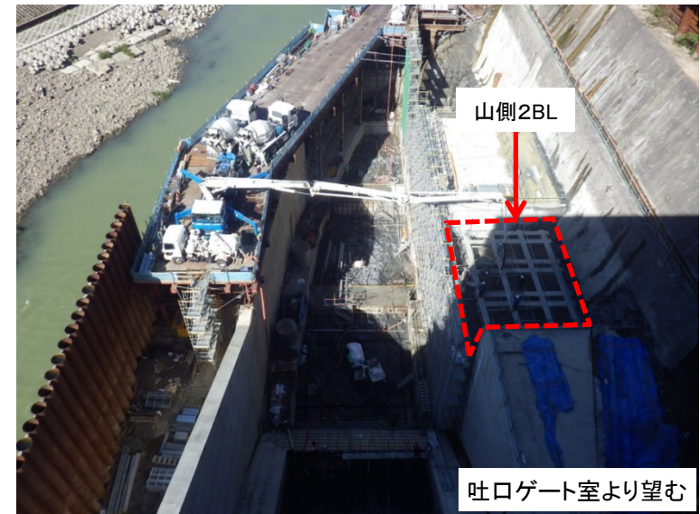
10月22日 山側2BLコンクリート打設
