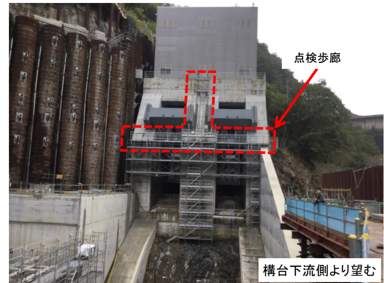
10月9日 点検歩廊設置完了
