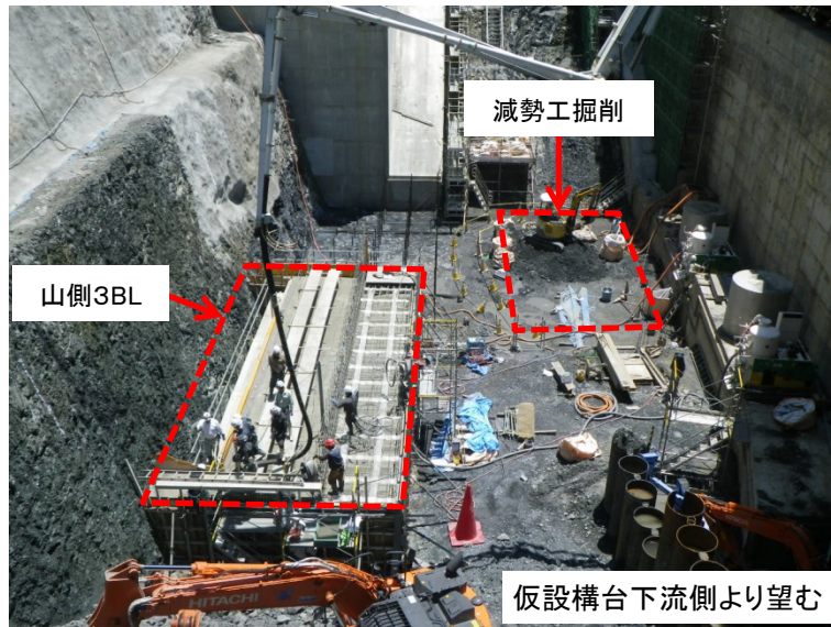
6月4日 減勢工掘削および山側3BLコンクリート打設
