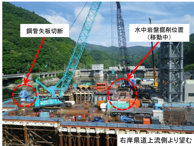
6月18日 掘削機による水中岩盤掘削、鋼管矢板切断
