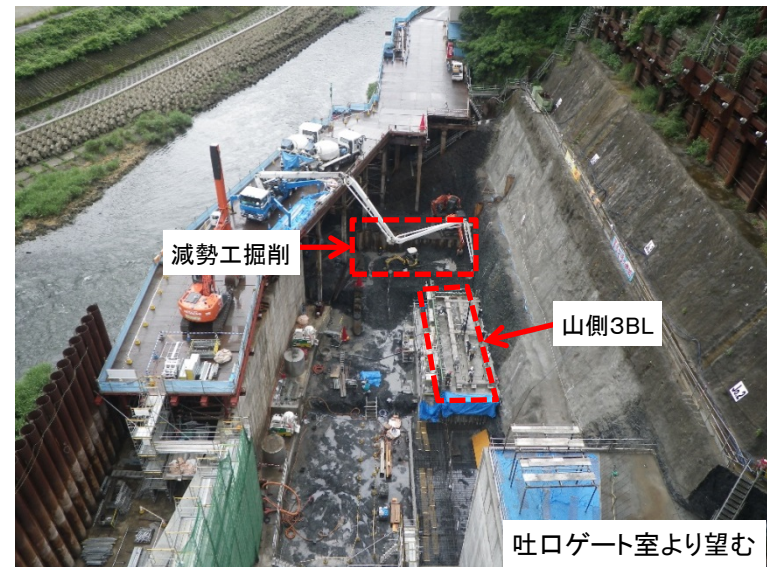
6月11日 減勢工掘削および山側3BLコンクリート打設
