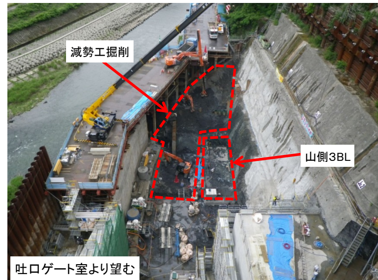
5月28日 減勢工掘削、山側3BL鉄筋組立
