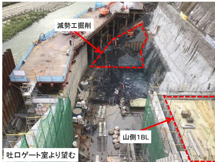
5月21日 減勢工掘削、山側1BL養生
