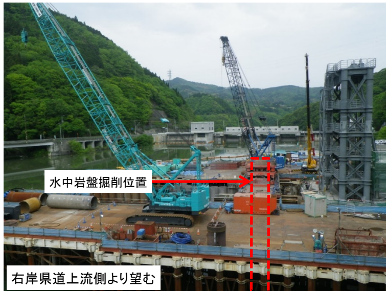
5月7日 掘削機による流入水路掘削
