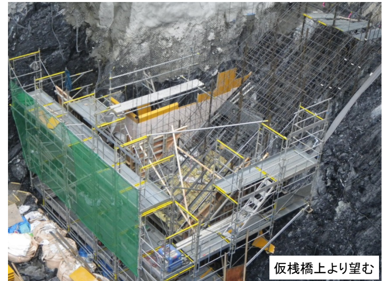
3月12日 山側1BL型枠組立
