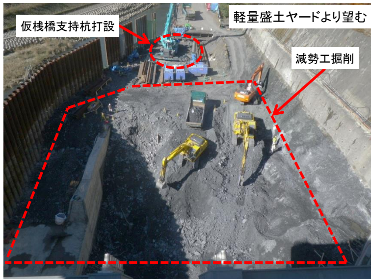
12月4日 減勢工掘削および仮棧橋支持杭打設
