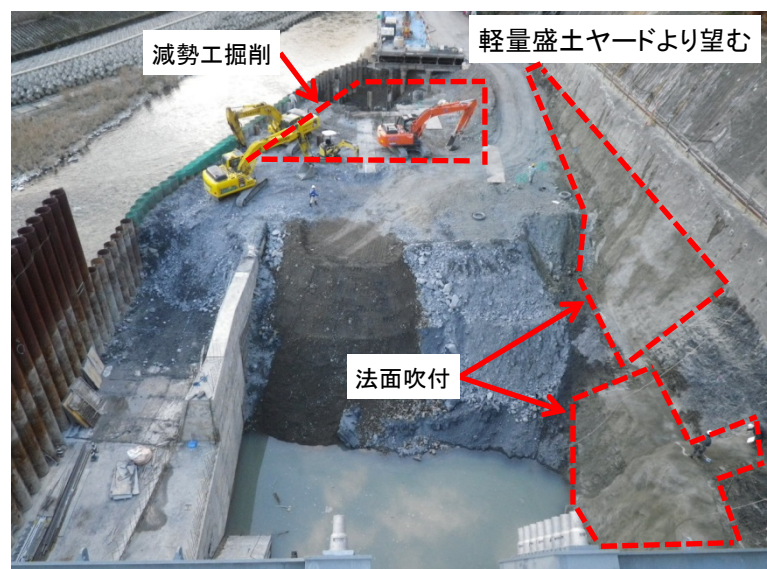
12月25日 減勢工掘削および法面吹付
