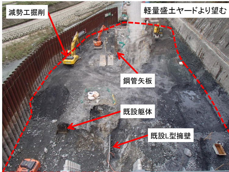
11月6日 減勢工掘削作業
