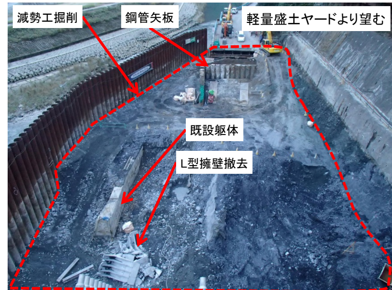
11月13日 減勢工掘削および既設L型擁壁撤去作業
