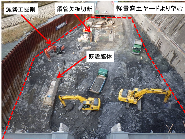
11月20日 減勢工掘削および鋼管矢板切断撤去作業
