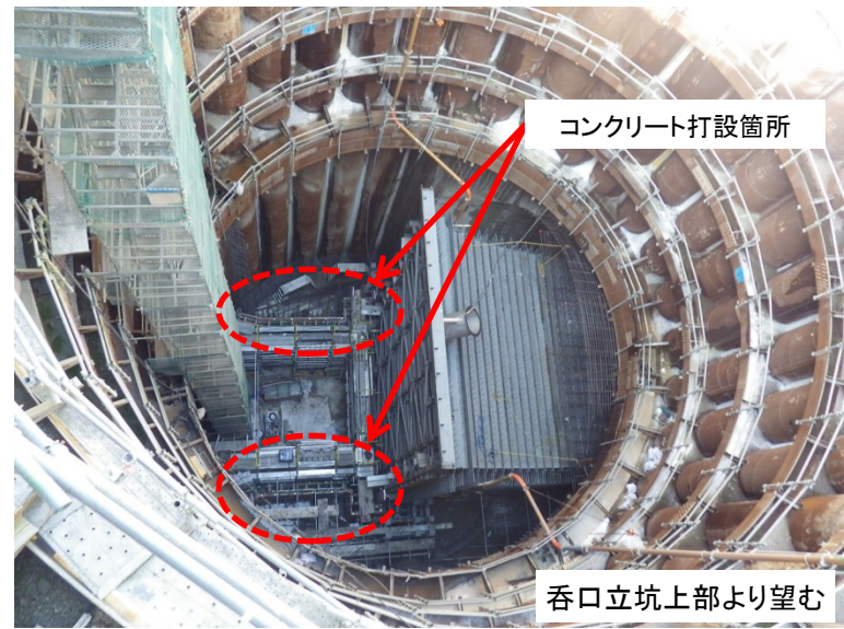
1月30日 27リフト中3リフトのコンクリート打設完了
