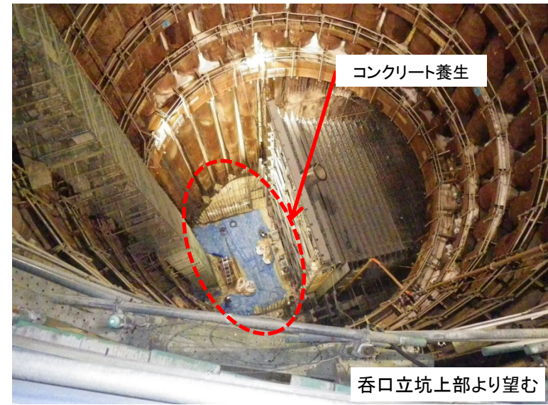
1月16日 27リフト中1リフトのコンクリート打設完了
