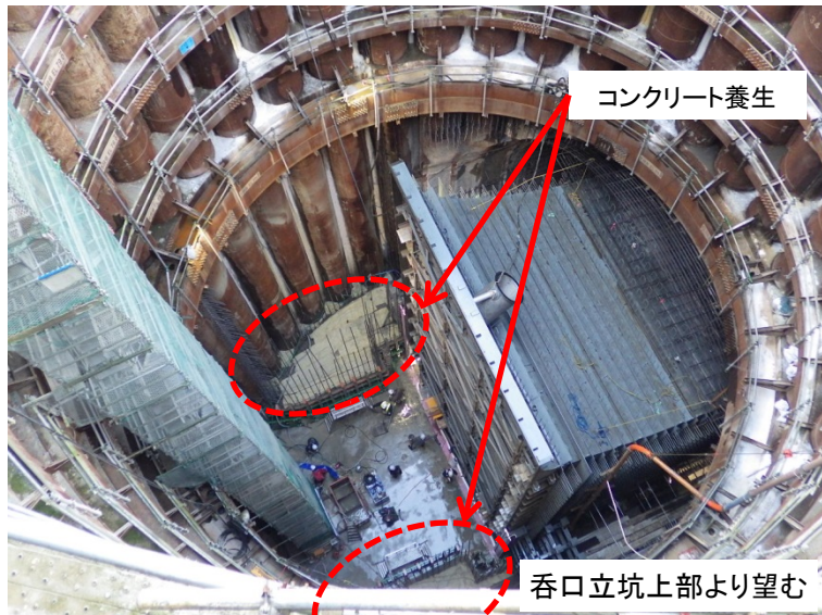
1月23日 27リフト中2リフトのコンクリート打設完了
