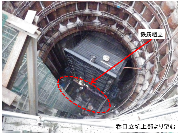
1月10日 27リフト中1リフトの鉄筋組立
