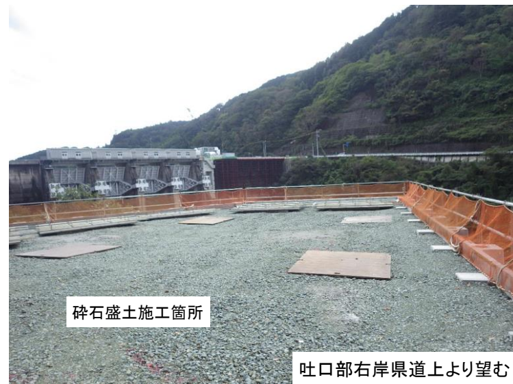
10月10日 軽量盛土工上部整備
