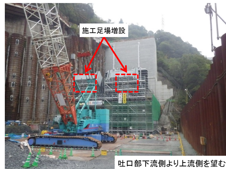
10月24日 施工足場増設
