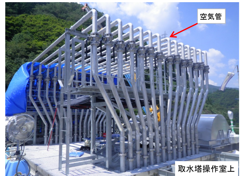
8月22日 空気管据付完了
