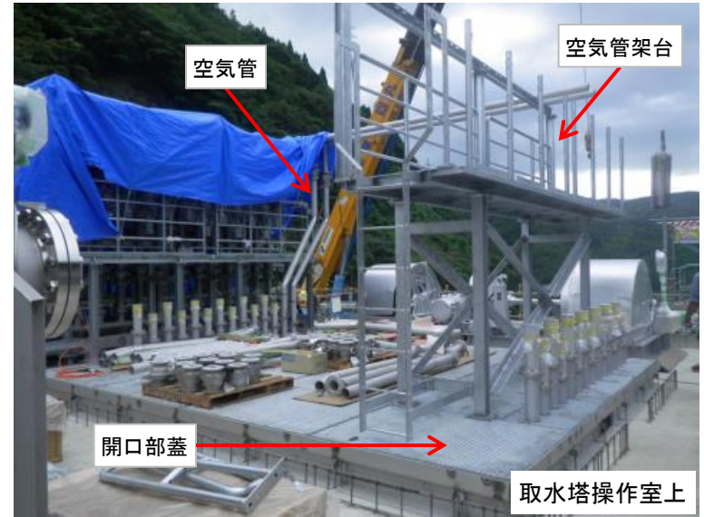
8月8日 付属設備据付
