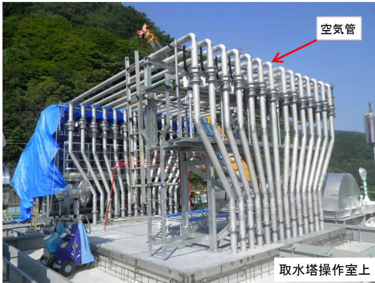
8月15日 空気管据付
