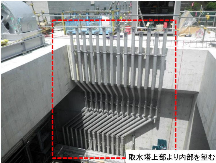
7月25日 空気管据付
