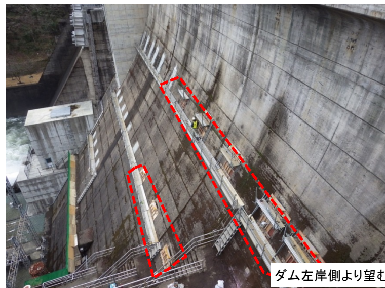
2月27日 下流側仮設構台支持杭撤去跡の補修
