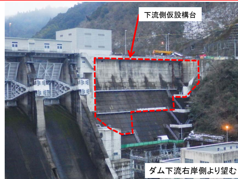
2月13日 下流側仮設構台撤去(95%)
