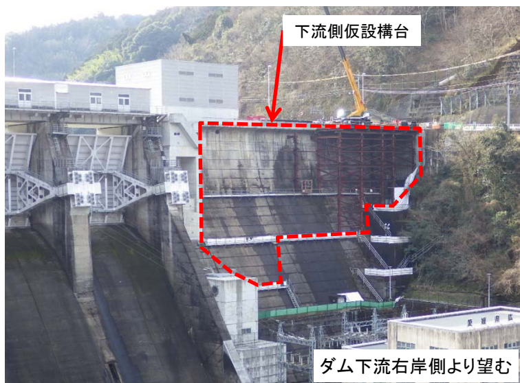
2月6日 下流側仮設構台撤去(60%)
