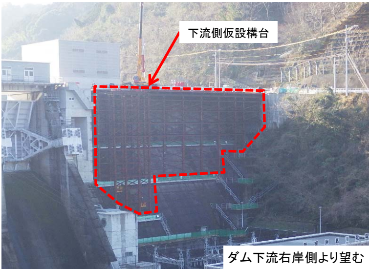
1月23日 下流側仮設構台撤去(12%)
