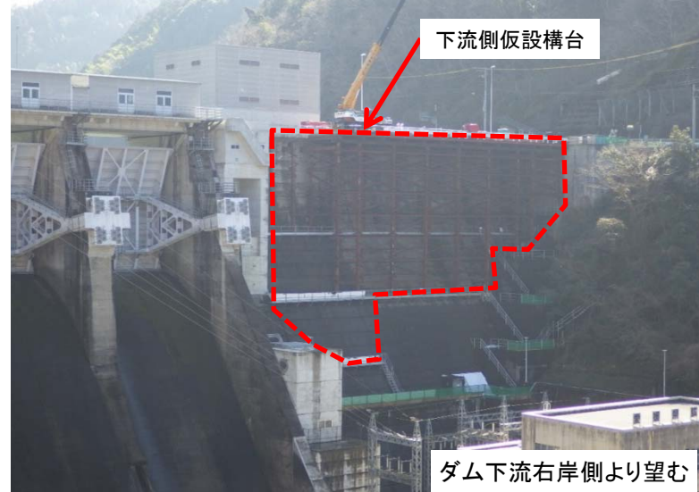
1月30日 下流側仮設構台撤去(30%)
