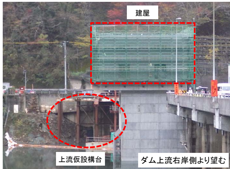
12月5日 建屋の防水、仕上作業、構台撤去(95%)
