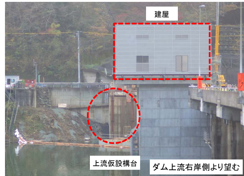
12月12日 足場解体作業、構台撤去(98%)
