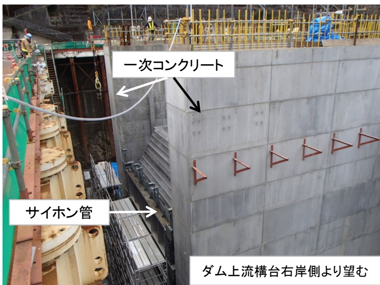
2月15日 水中部・気中部二次コンクリート打設
