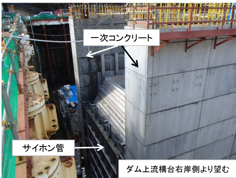
2月1日 水中部二次コンクリート打設
