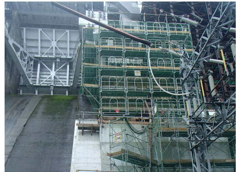
9月8日 低水放流バルブ室構築
