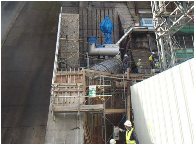
7月7日 ゲート室構築
