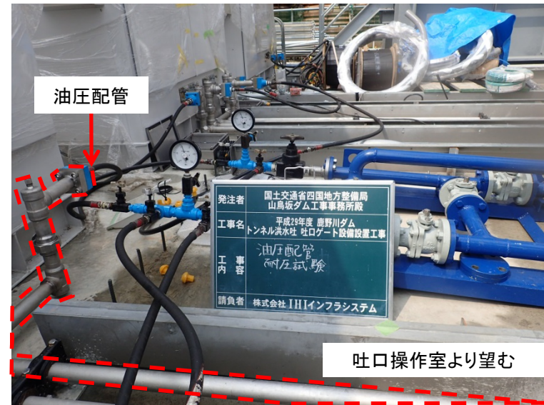
8月14日 油圧配管(耐圧試験)
