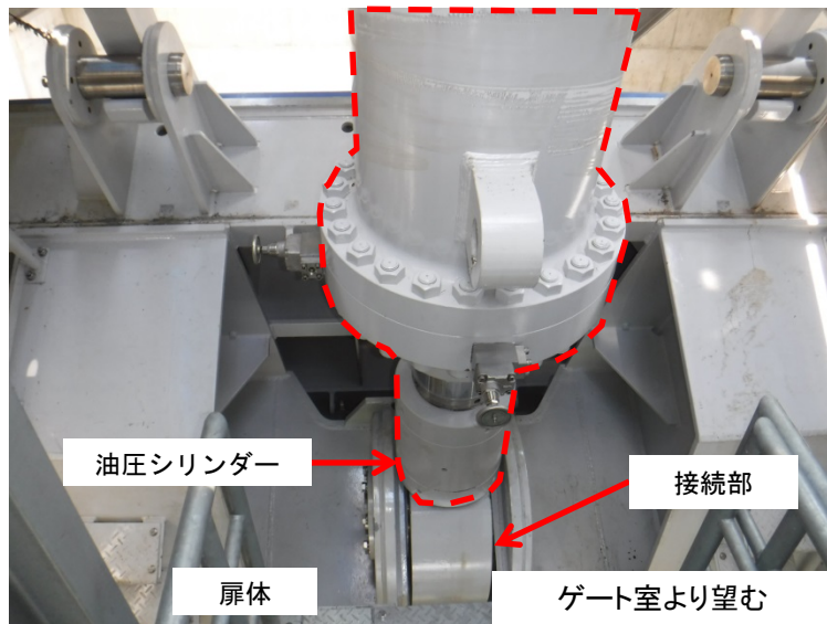
8月21日 扉体と開閉装置(油圧シリンダー)の接続
