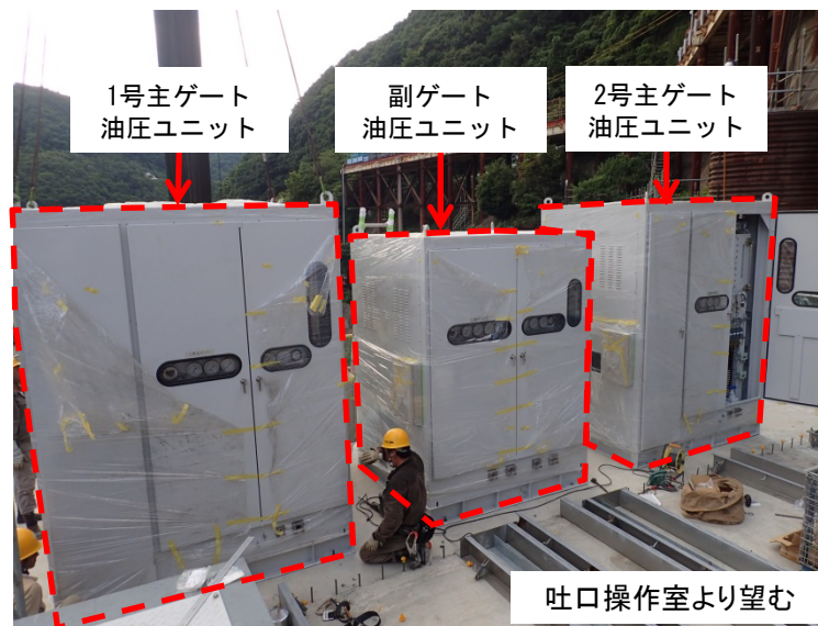
7月24日 開閉装置(油圧ユニット)設置
