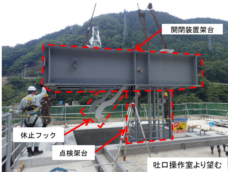
7月17日 主ゲート開閉装置設置
