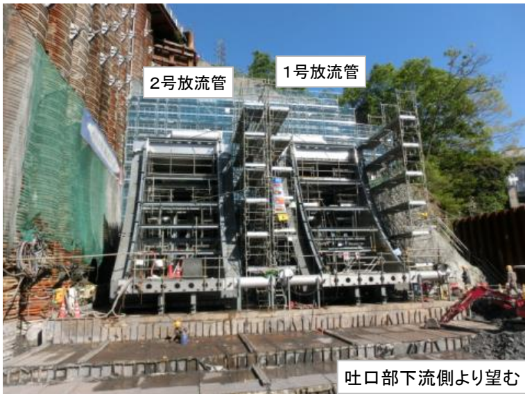
5月9日 放流管据付完了
