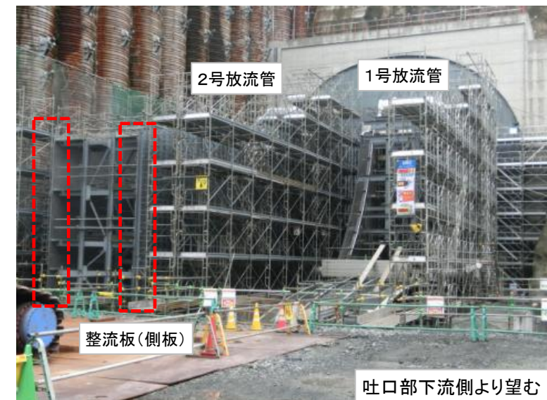
5月30日 2号整流板(側板)設置
