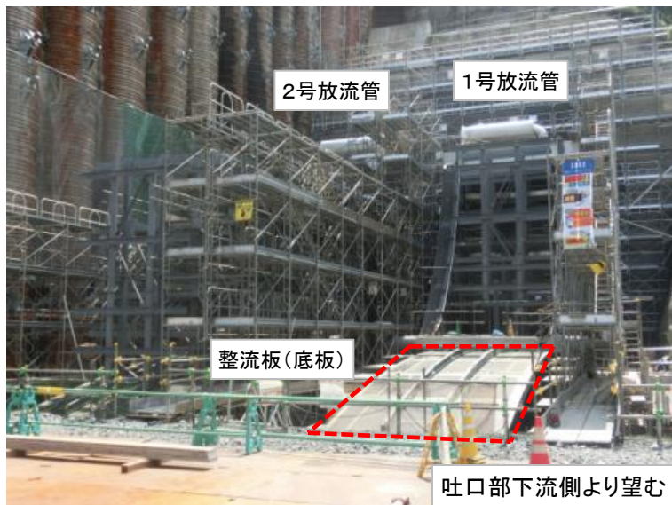
5月23日 整流板(底板)据付
