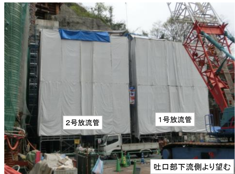
4月11日 2号放流管組立
