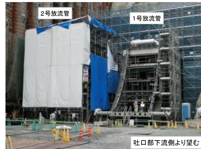
4月25日 1号放流管足場解体
