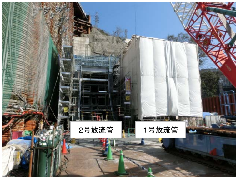
3月22日 1号放流管溶接
