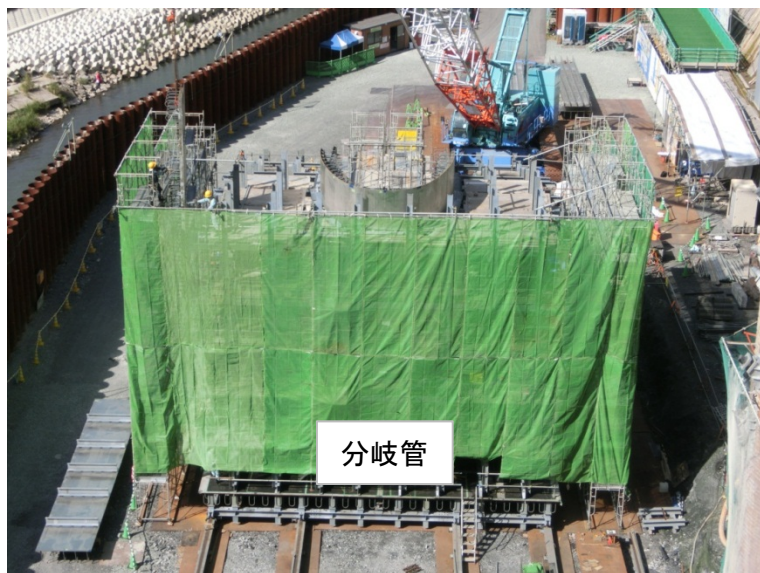
11月2日 分岐管組立
