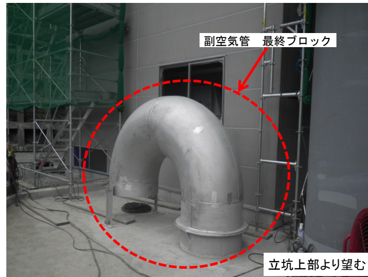
6月4日 副空気管据付完了
