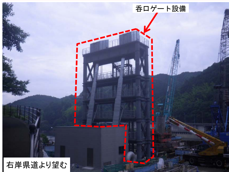
6月11日 機械設備全ての据付完了
