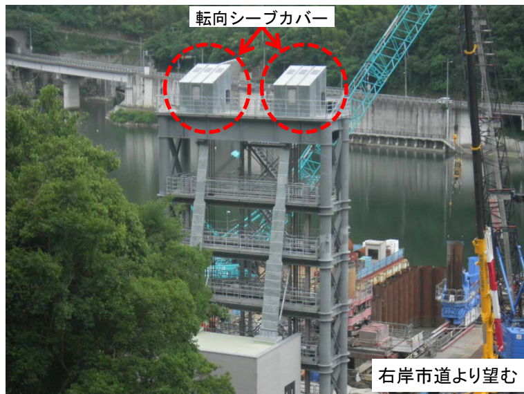
6月4日 転向シーブカバー据付完了
