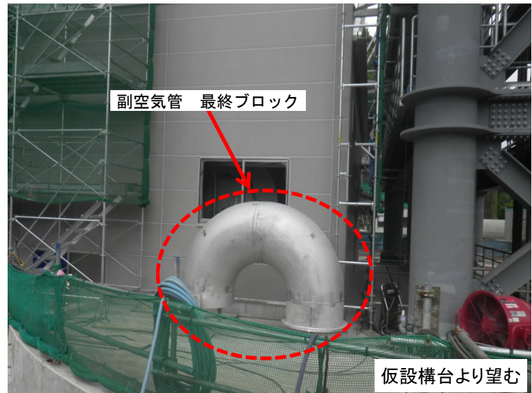
5月28日 副空気管最終ブロック据付
