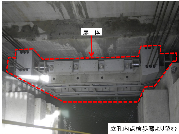
5月7日 立孔内注水 → 扉体確認
