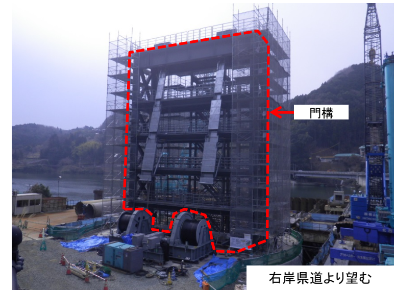
2月26日 門構組立
