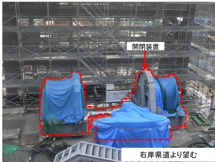
2月5日 開閉装置組立
