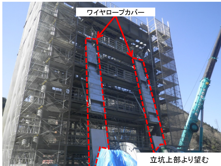
2月19日 開閉装置(ワイヤーロープカバー)組立
